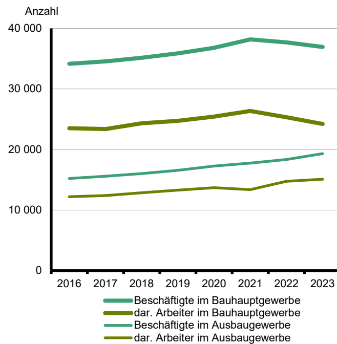
Beschäftigte im Bauhaupt- und Ausbaugewerbe seit 2016 im Land Brandenburg
